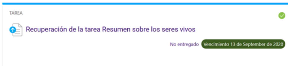
Figura 6: Tarea
