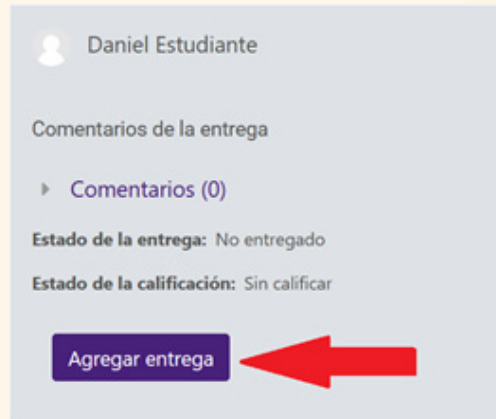
Figura 7: Agregar Entrega
