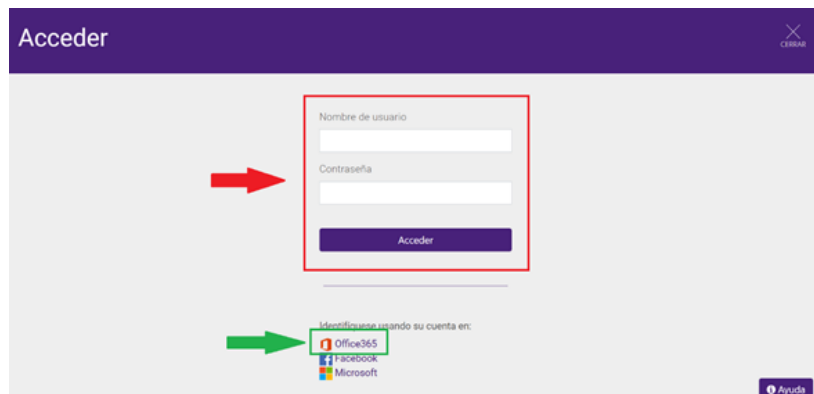
Figura 2: Acceder
